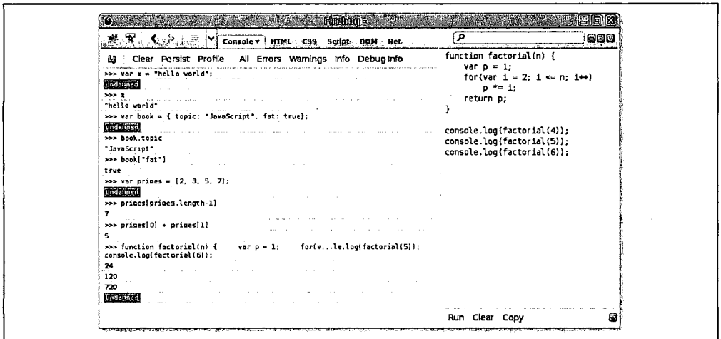
图1-1: Firebug控制台
