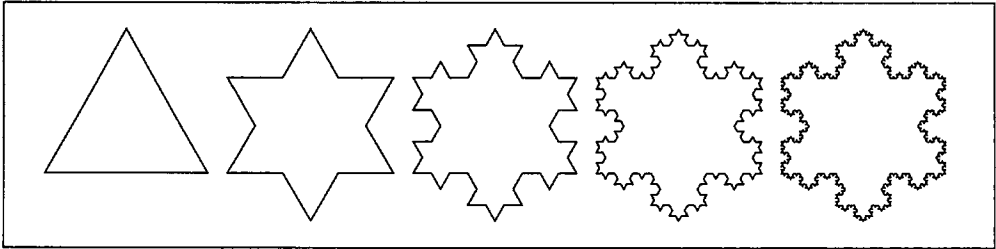
图21-8：科赫雪花
