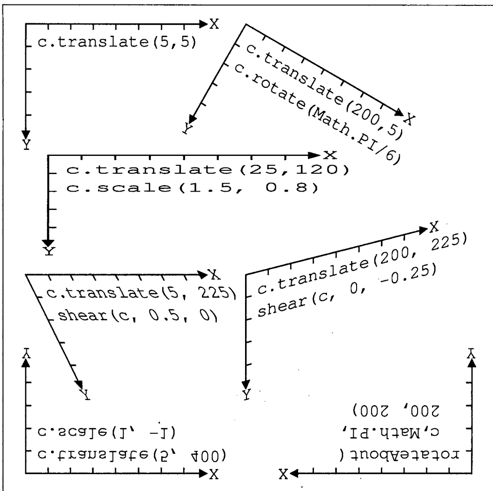
图21-7: 坐标系变换
