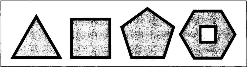
图21-6: 规则多边形
